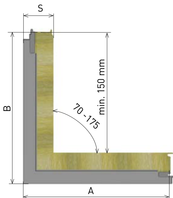
Rys. 2.5: Narożnik w kształcie L
