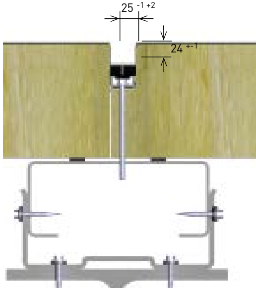
Rys. 1.2: Element fasadowy QO B – montaż poziomy
