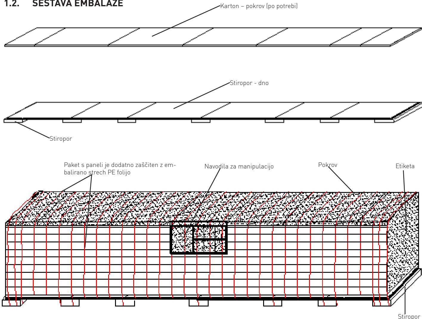
Slika 2: Elementi embalaže Trimoterm panelov
